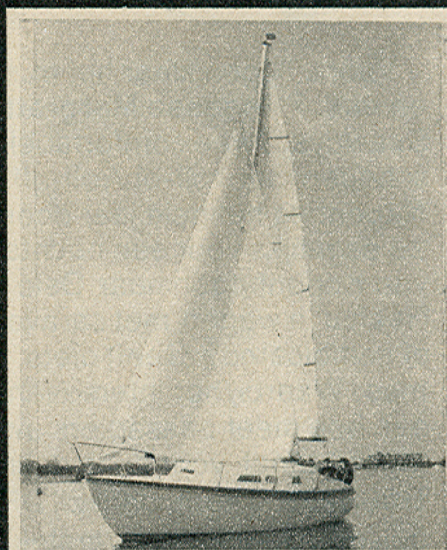
SUPER DAIMIO. Zeewaardig onkenterbaar pol. zeilj met 5 slaappl., afm. 8.40 x 2.90 m, diepg. 1.25 m, gewicht 3000 kg, zeilopp. 34 m 2 , met 11 pk Gouach diesel. Vaarklaar f52.950,— inkl. 16% btw.
